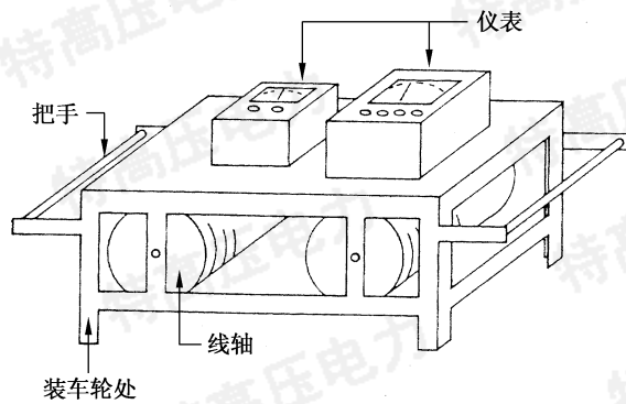
图 21 测试小车
