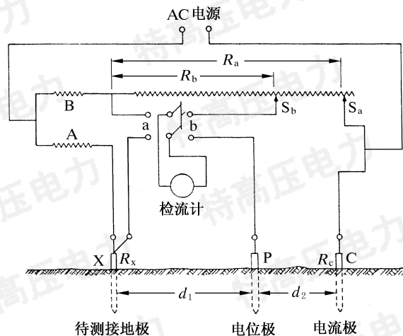
图 15 双平衡电桥
