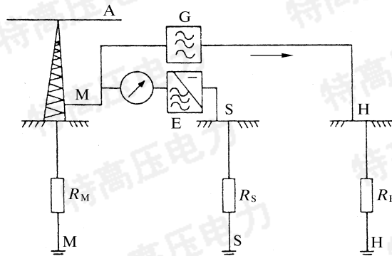
M—铁塔;A—架空地线;S—电位极; R_M —铁塔接地电阻;H—电流极; R_S —电位极接地电阻;G—高频发生器; R_H —电流极接地电阻;E—高频接收器
