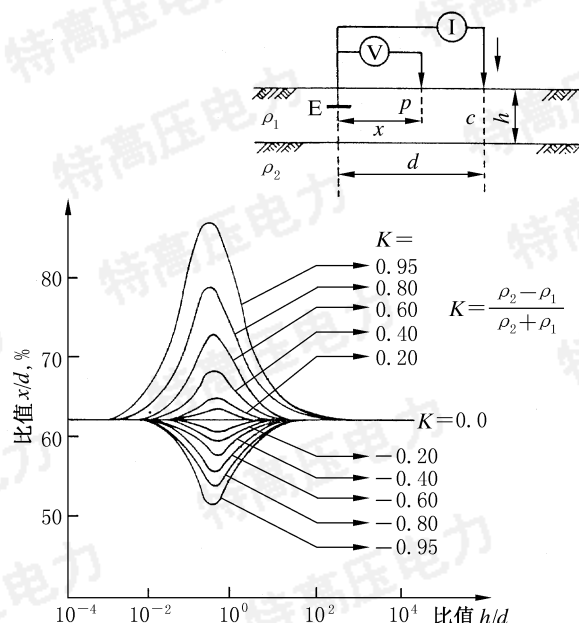
图 10 两层土壤时电位极的所需位置
