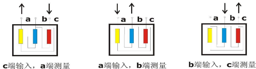
图 5 内连接△接线
