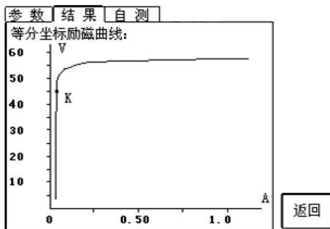
图 2.16 励磁曲线界面
