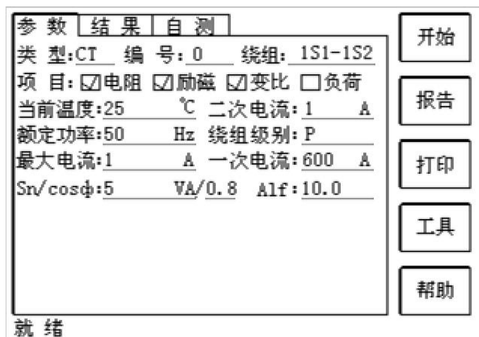
图 2.3 基本参数设置界面
